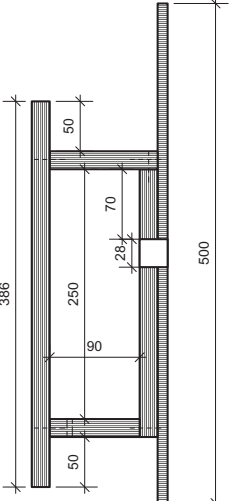
Section B-B 1:4
