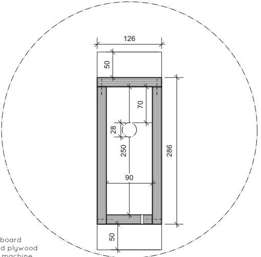
Section A-A 1:4
